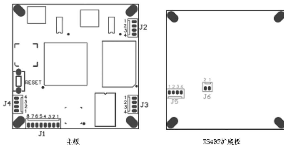
图 1-1 IP5150 接口
